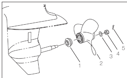
Рис. 6 Гребной винт
