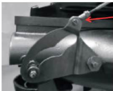
А - ГАЙКА РЕГУЛИРОВКИ ТРОСА ПЕРЕКЛЮЧЕНИЯ ПЕРЕДАЧ
